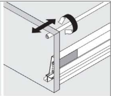
Lutningsjustering
