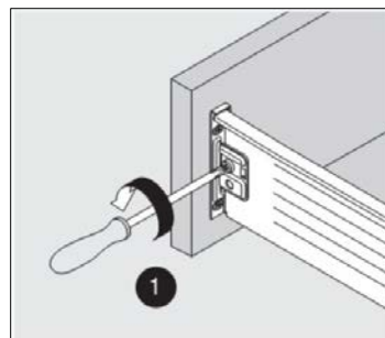
Höjdjustering (B)
