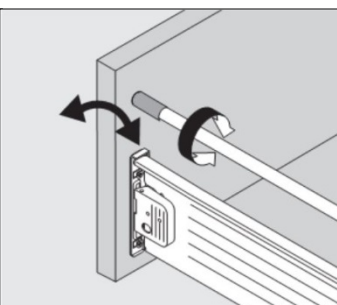
Lutningsjustering
