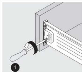
Höjdjustering (A)
