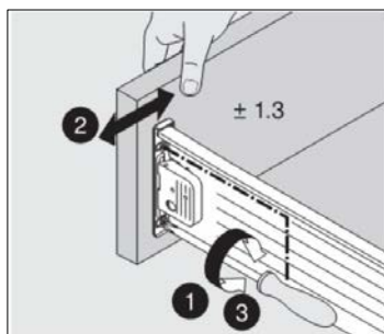
Sidjustering (A)
